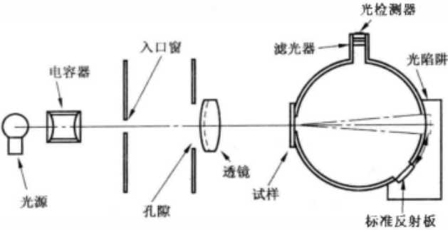
图 1 雾度计示意图
